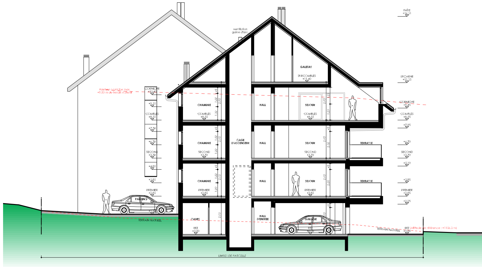
COUPE TRANSVERSALE
